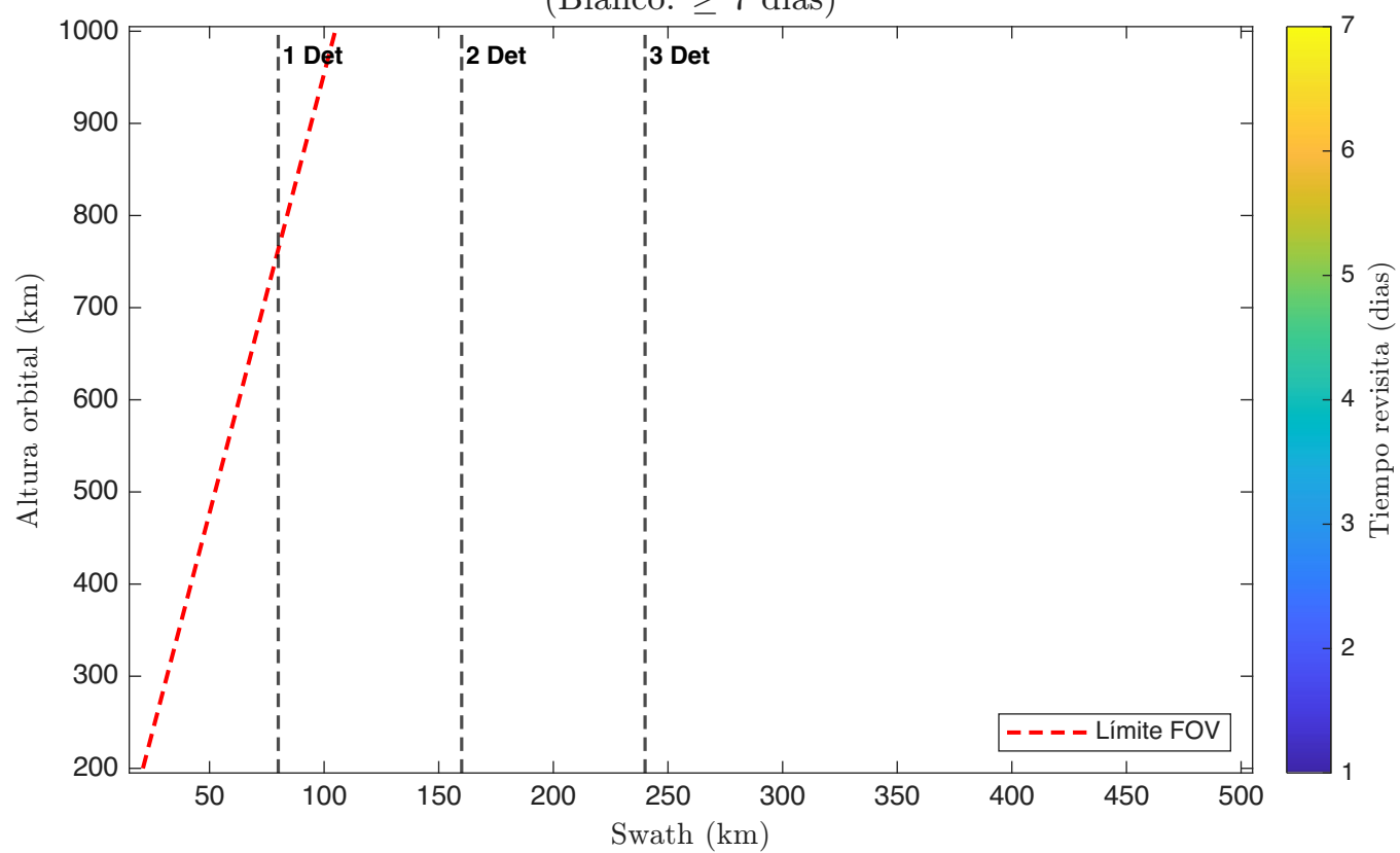
Tiempo Revisita - 1 Satellite(s); 2 Telescopio(s): Cassegrain; Detector 3 (Blanco: \geq 7 dias)
